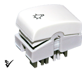
3254 Módulo Interruptor Pulsador Minuteria 10A/250V (Lâmpada Gravada)
